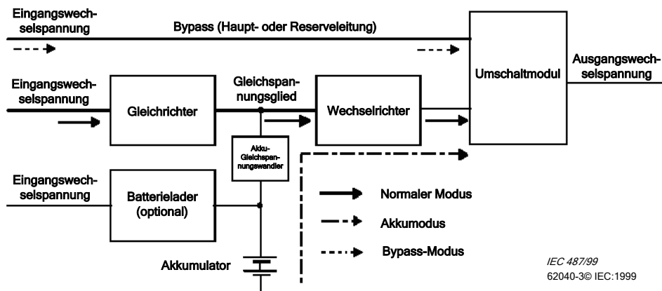
Abbildung 5 – USV-Topologie mit Online-Doppelwandlung aus IEC 62040-3 Blockdiagramm mit vier Wandlerblöcken
